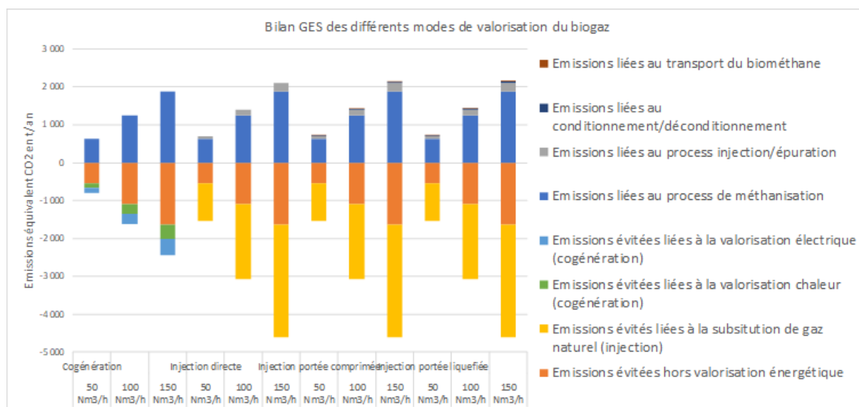
Comparaison du bilan GES d'unités de méthanisation de 50, 100 et 150 Nm 3 /h en fonction d'une valorisation par cogénération, injection directe ou injection portée
